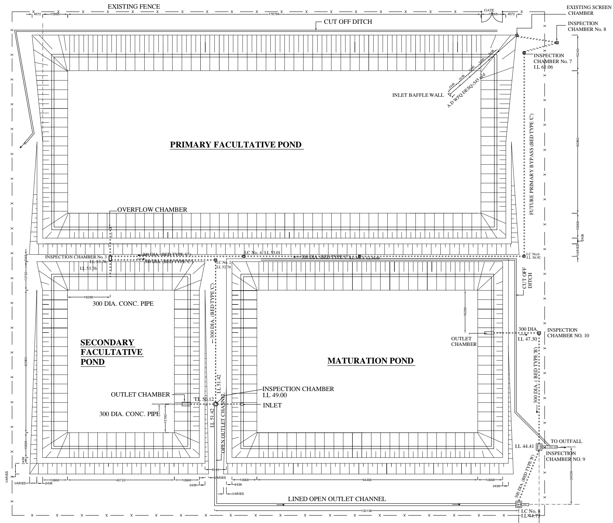
PLAN-OXIDATION PONDS
